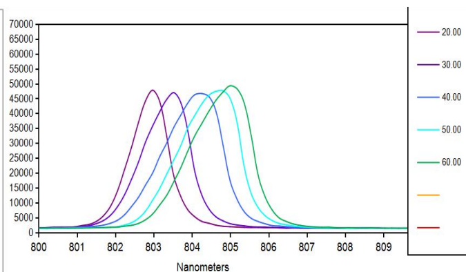
光谱曲线
