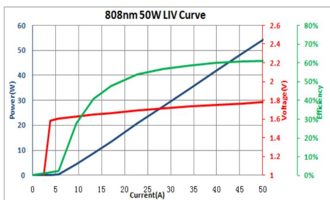
LIV 曲线
