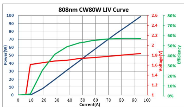
LIV 曲线
