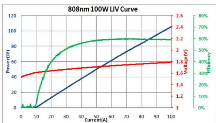
LIV 曲线
