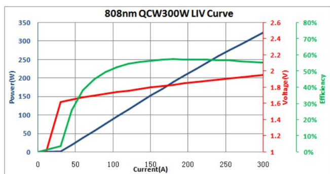
LIV 曲线
