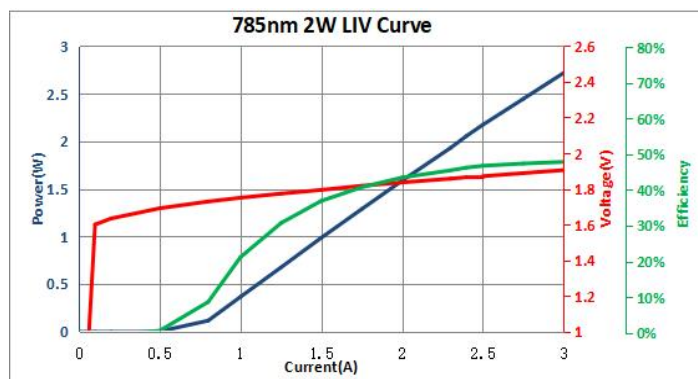
LIV 曲线
