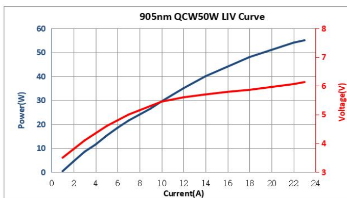
LIV 曲线
