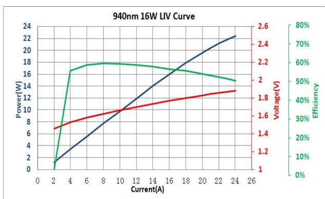
LIV 曲线
