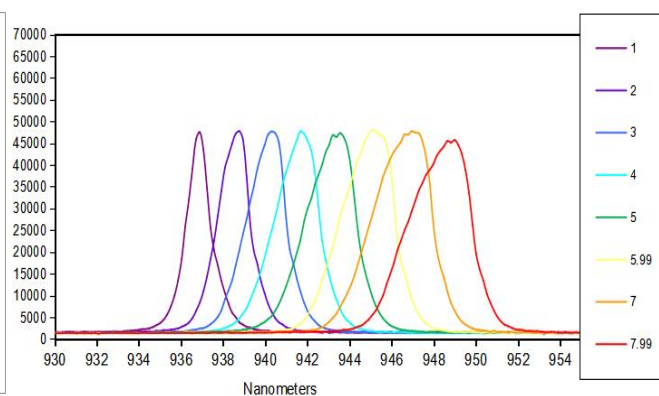
光谱曲线
