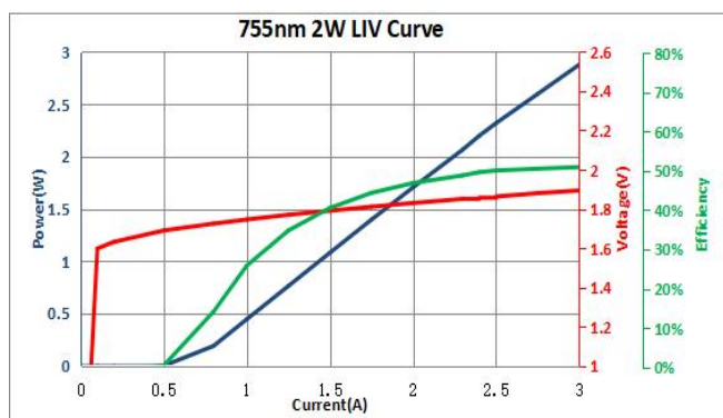
LIV 曲线
