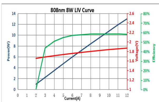
LIV 曲线
