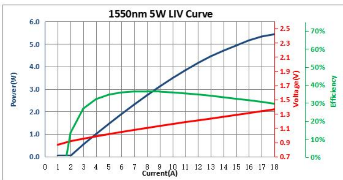
LIV 曲线
