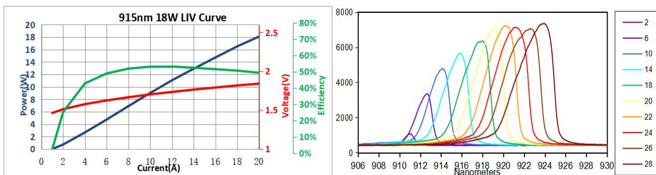
LIV 曲线
