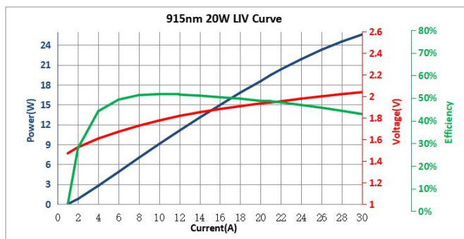
LIV 曲线
