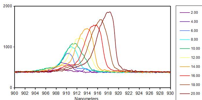
光谱曲线
