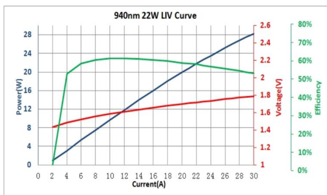
LIV 曲线
