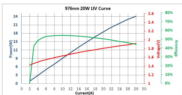
LIV 曲线
