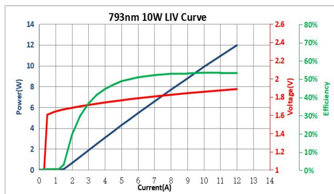
LIV 曲线
