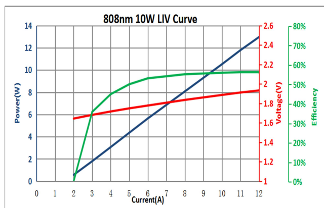
LIV 曲线
