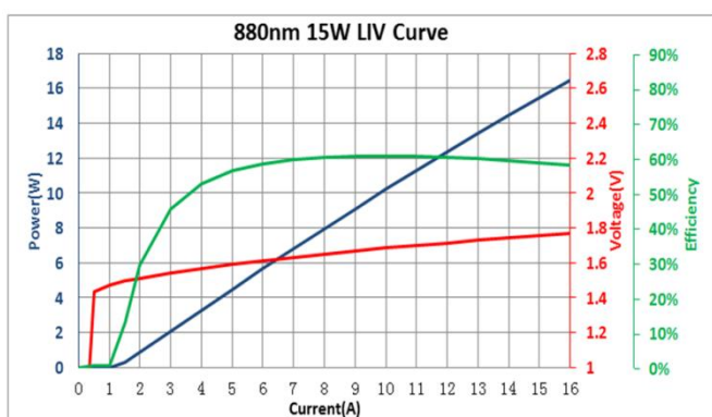
LIV 曲线
