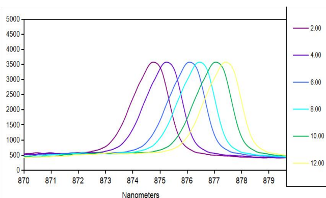
光谱曲线
