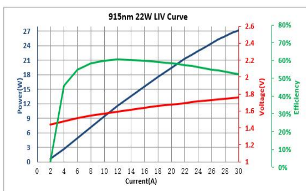
LIV 曲线
