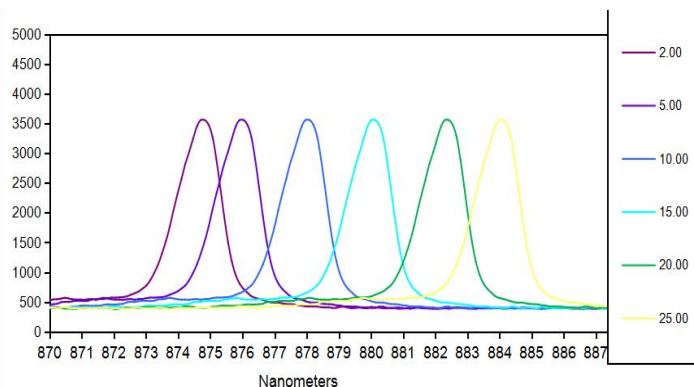
光谱曲线
