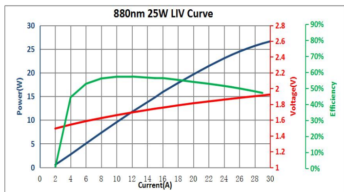
LIV 曲线
