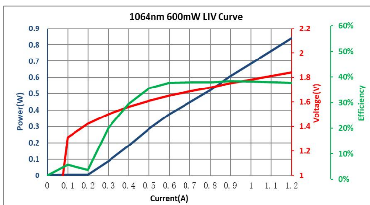
LIV 曲线
