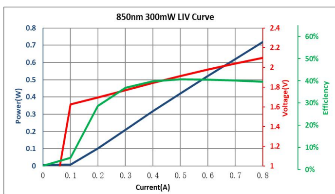
LIV 曲线
