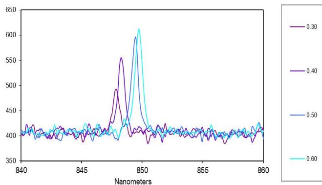
光谱曲线
