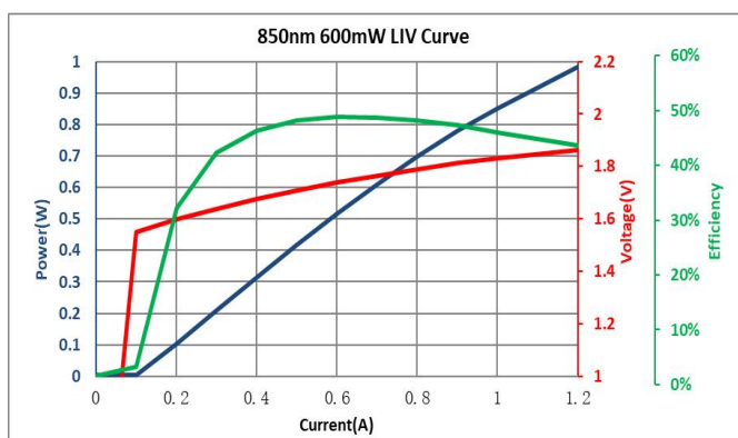
LIV 曲线
