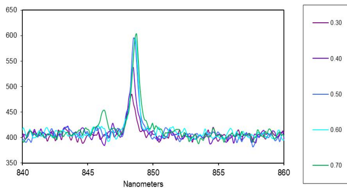
光谱曲线
