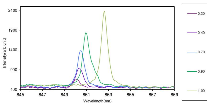
光谱曲线
