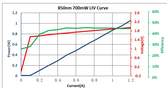
LIV 曲线
