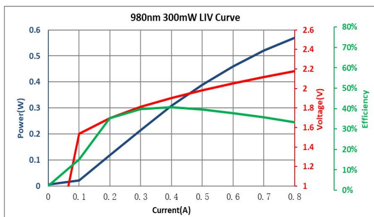
LIV 曲线
