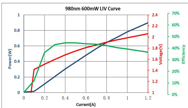
LIV 曲线
