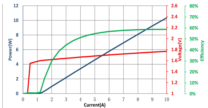
LIV 曲线
