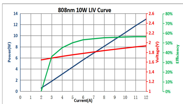
LIV 曲线
