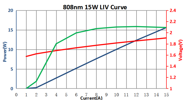
LIV 曲线
