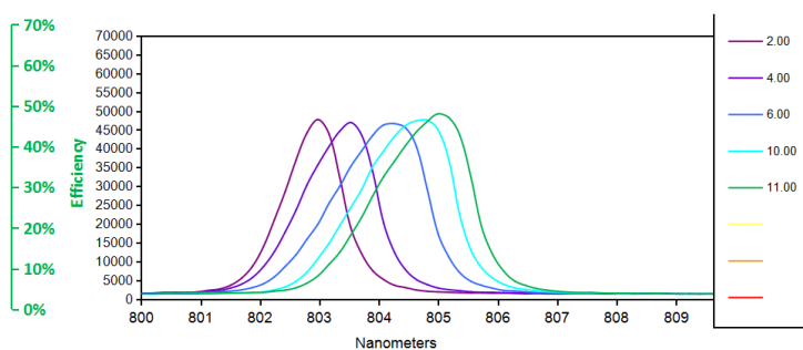
光谱曲线
