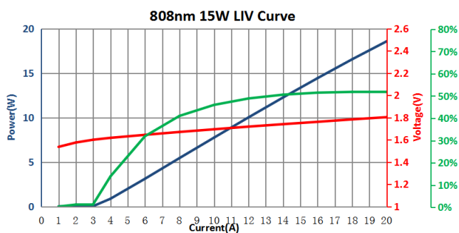
LIV 曲线
