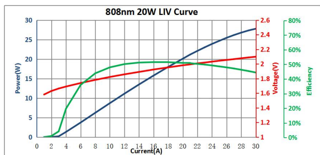
LIV 曲线
