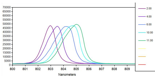
光谱曲线
