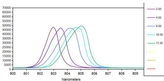
光谱曲线
