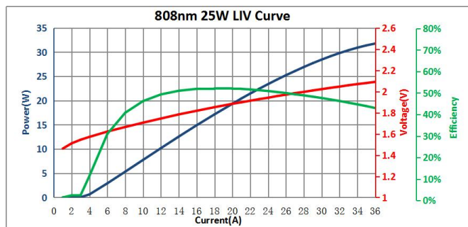
LIV 曲线
