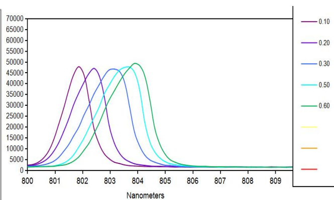
光谱曲线
