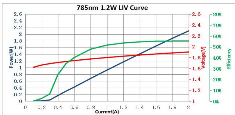
LIV 曲线
