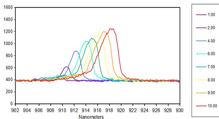
光谱曲线
