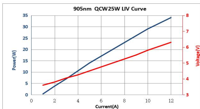
LIV 曲线
