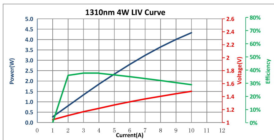
LIV 曲线
