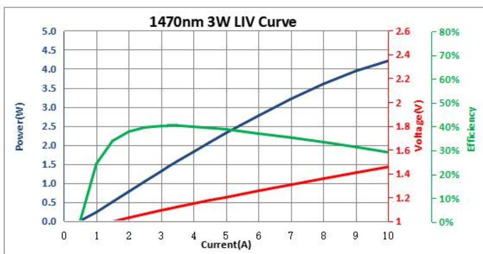
LIV 曲线
