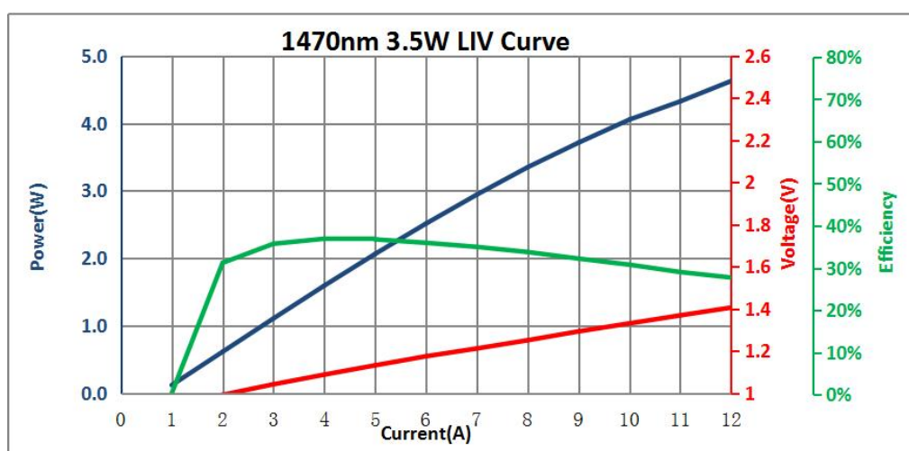
LIV 曲线
