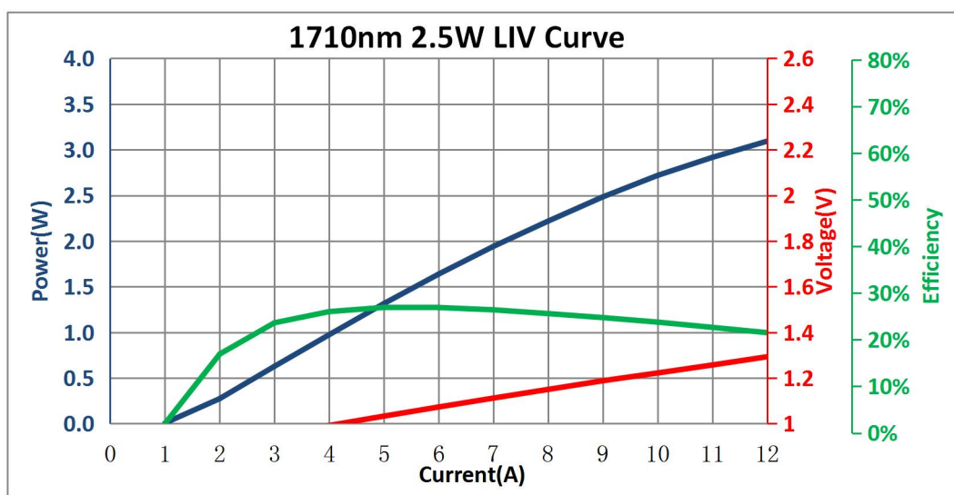
LIV 曲线
