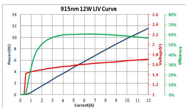
LIV 曲线
