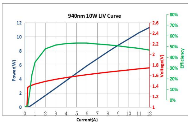
LIV 曲线
