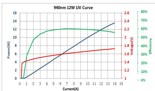
LIV 曲线
