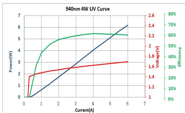
LIV 曲线
