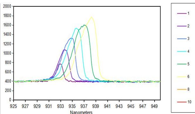
光谱曲线
