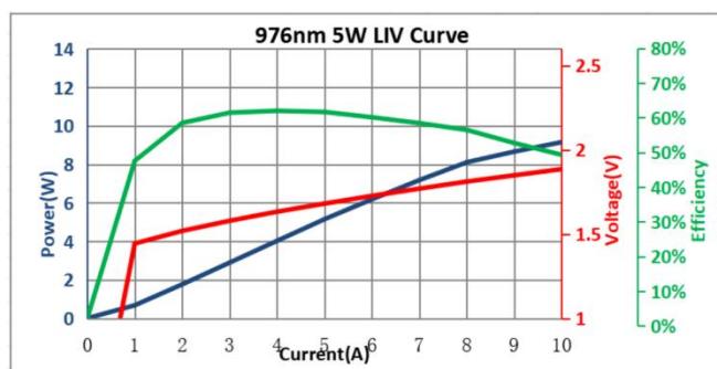
LIV 曲线
