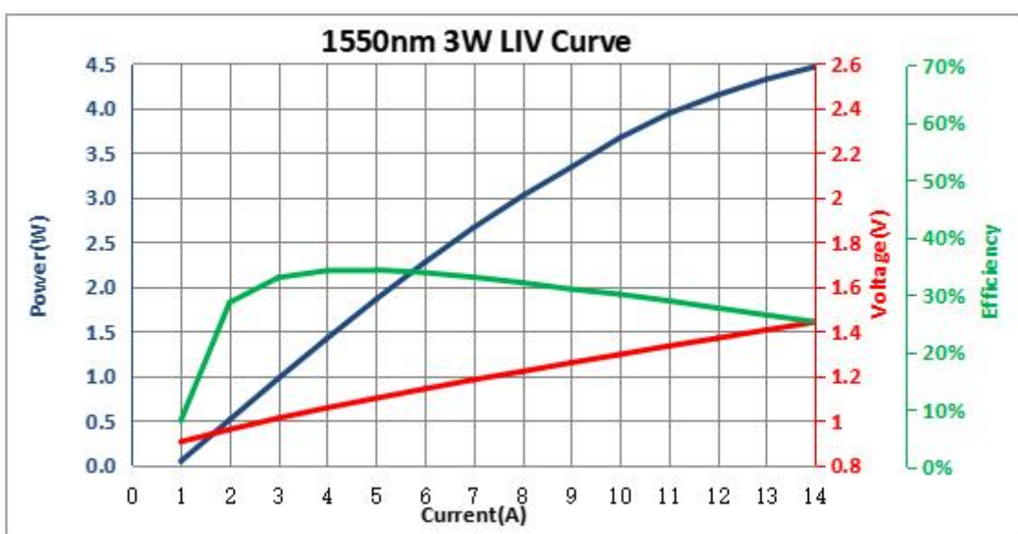
LIV 曲线
